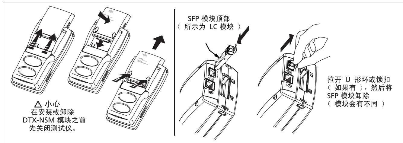
图 23. 安装和拆除网络模块和 SFP 模块
