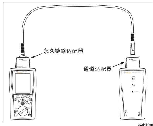
图 9. 双绞线基准连接
