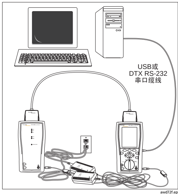
图 29. 用 PC 更新软件
