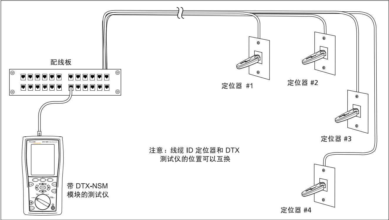
图 28. 利用可选件 LinkRunner 线缆 ID 定位器来识别链路
