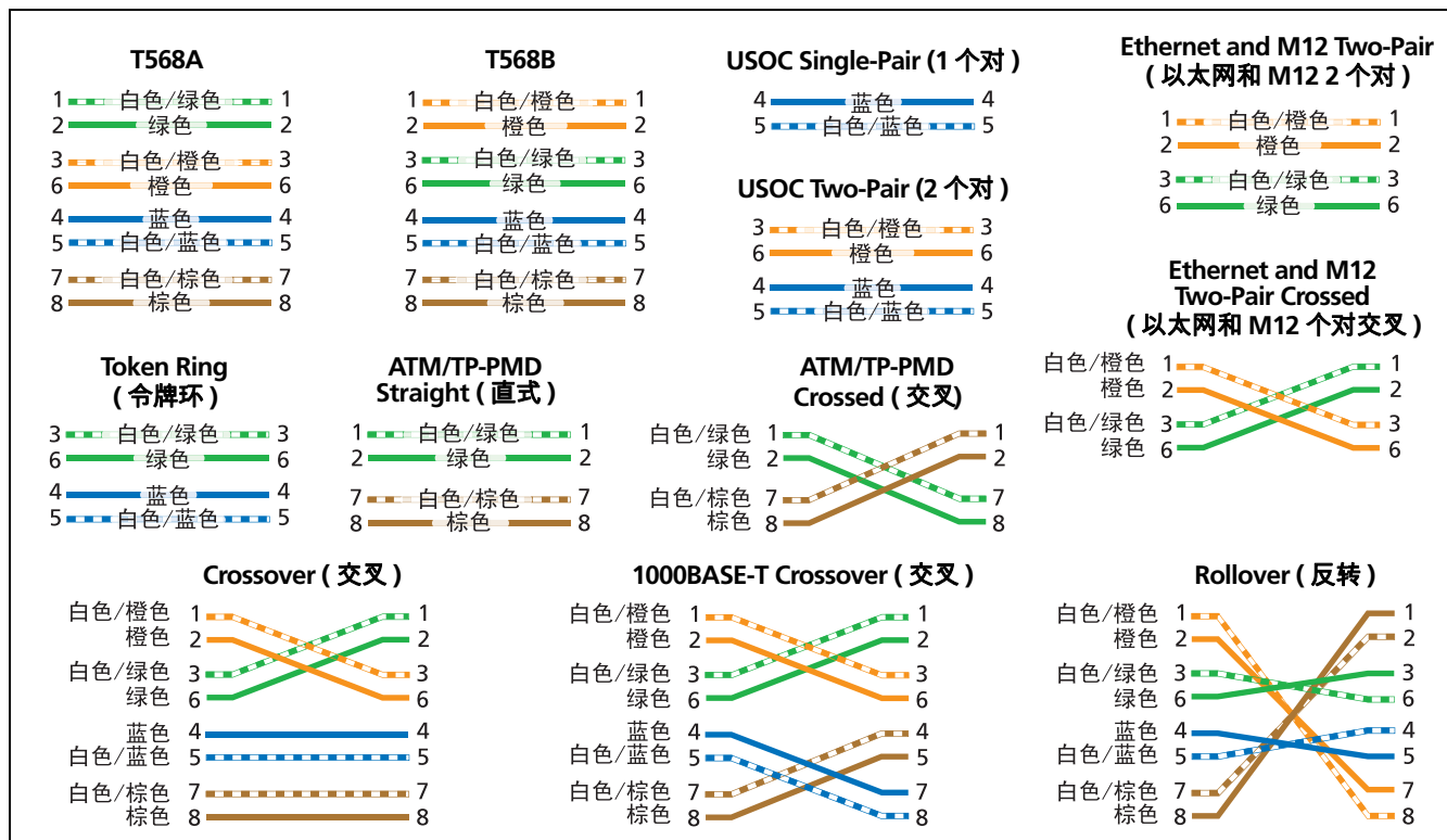
图 10. 插座配置
