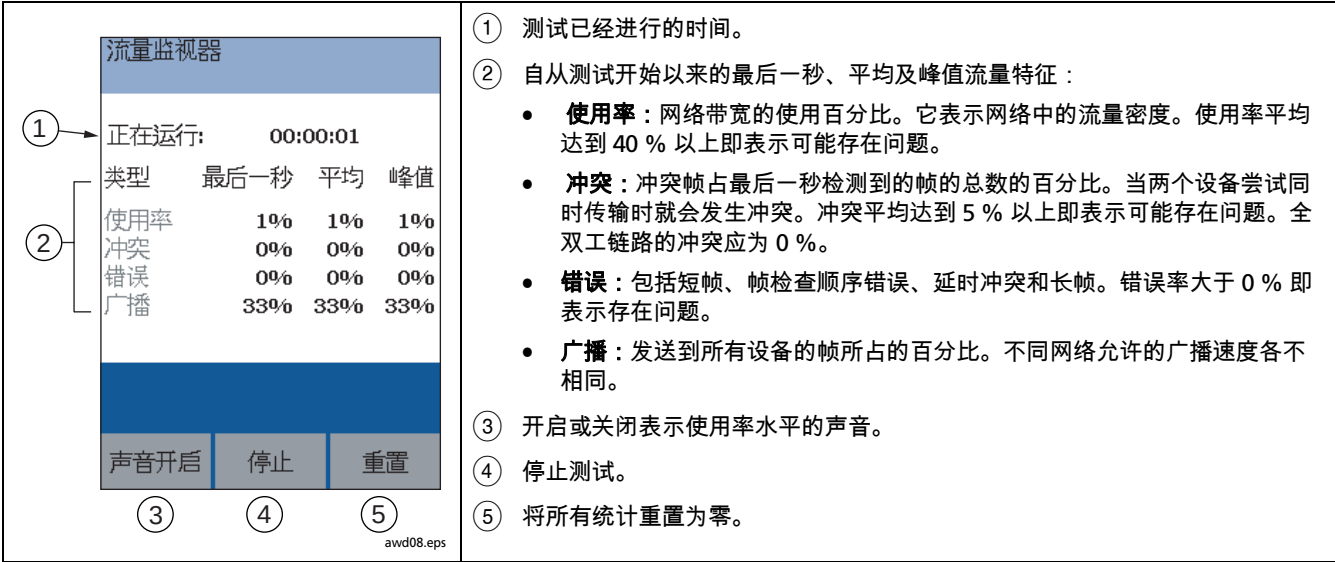
图 27. 流量监视器屏幕
