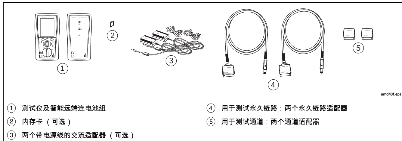
图 11. 认证双绞线布线所需的装置
