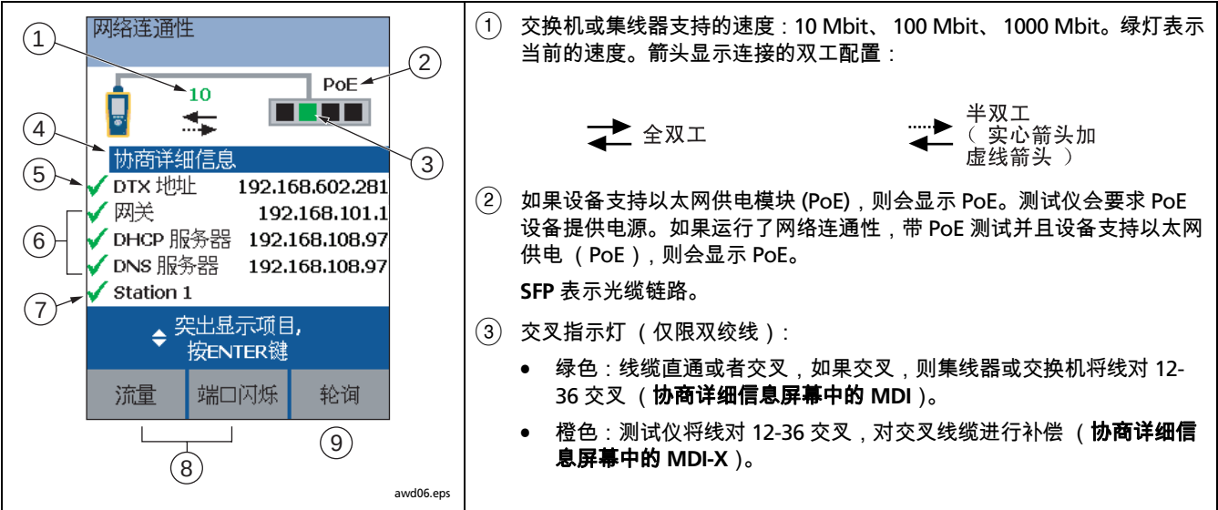
图 25. 网络连通性测试结果屏幕（以双绞线 DHCP 配置为例）
