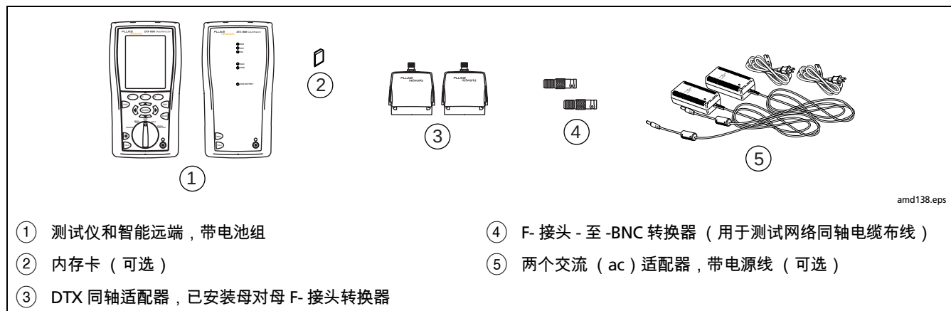
图 18. 同轴电缆布线认证设备
