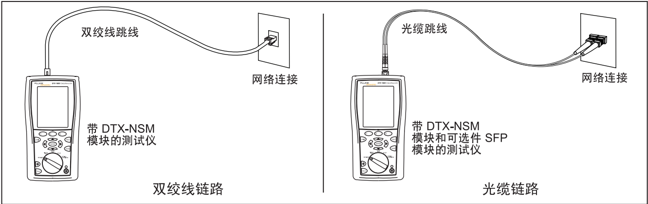
图 24. 网络测试连接
