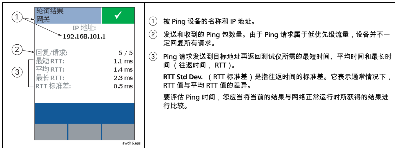
图 26. Ping 结果屏幕
